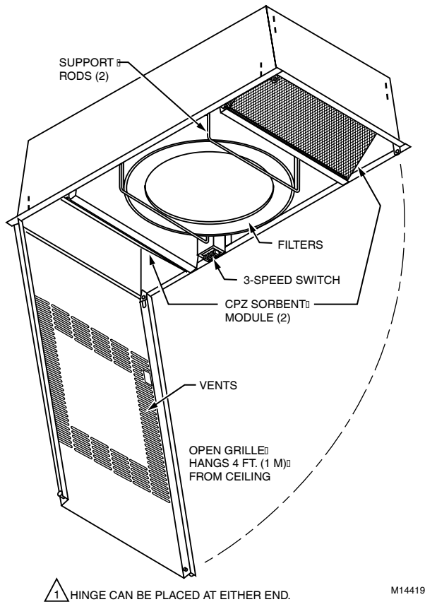
Fig. 8. Installing grille.
